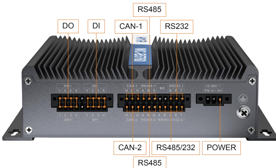
图 2-1 MIC-B5760 工控机正面接口标注图
