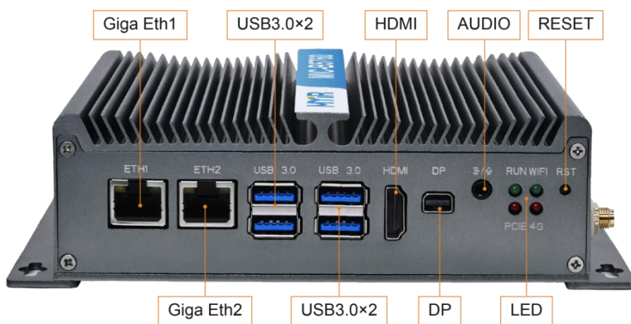
图 2-1 MIC-B5760 工控机正面接口标注图
