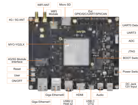
MYD-YG2LX开发板正面接口图
