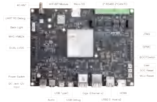
MYD-YM62X开发板正面接口图
